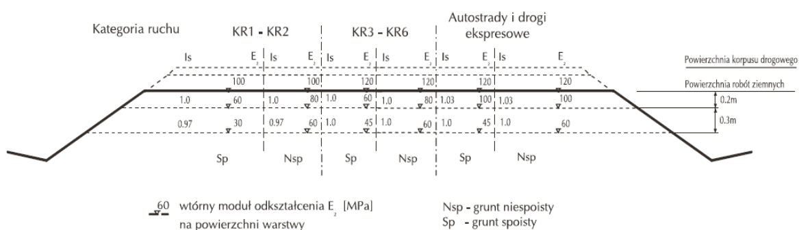
Wymagane parametry podłoża dróg w wykopach
